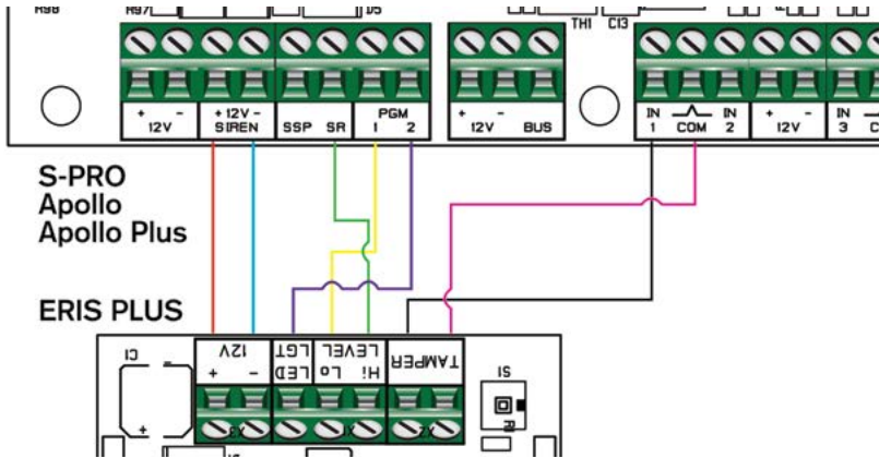
Συνδεσμολογία ERIS PLUS με πίνακες Sigma
